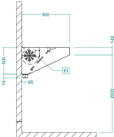
Zij aanzicht
